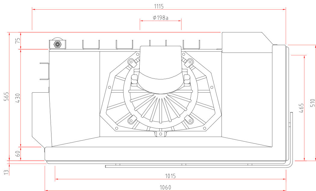
Draufsicht M 1:10
