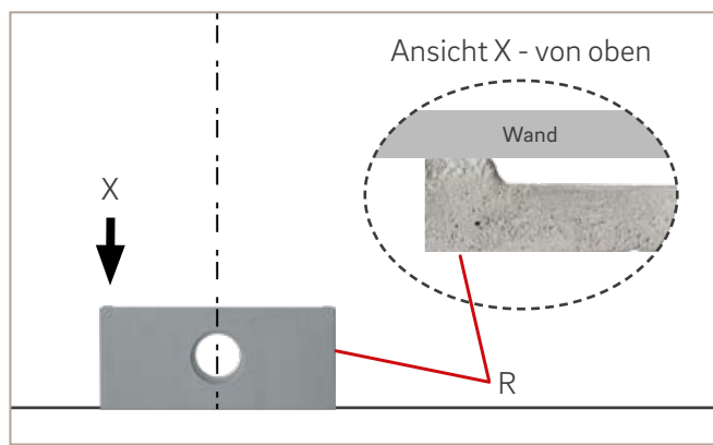
Abb.20: Rückwand 1 ausrichten
