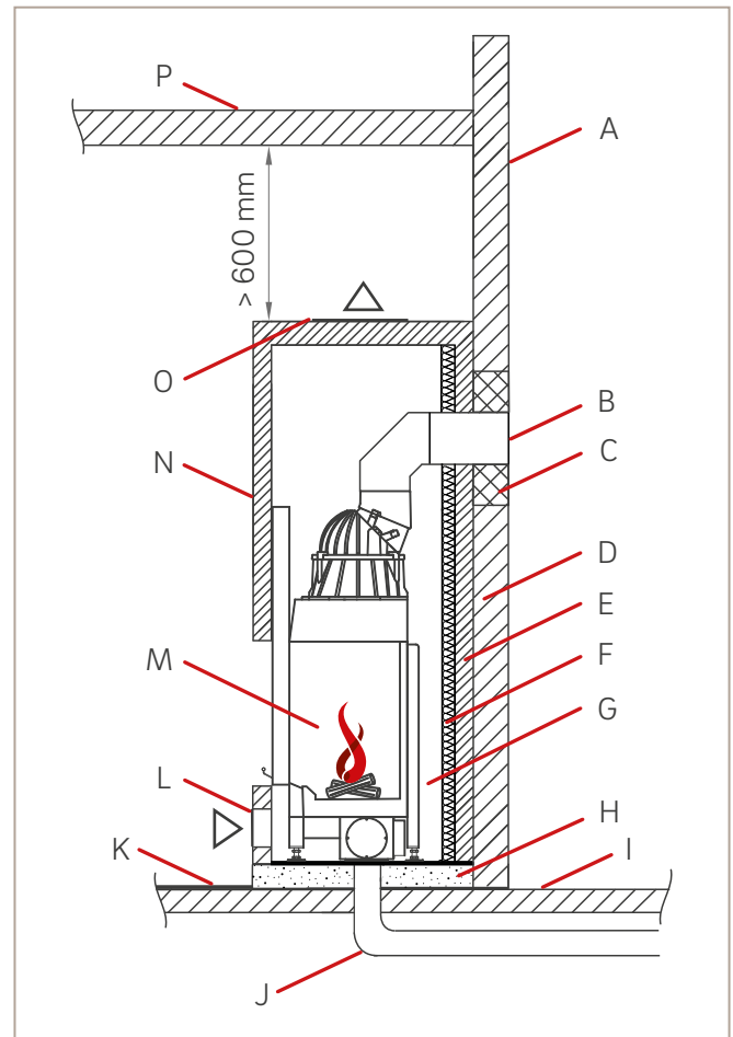
Abb. 73: Einbaubeispiel für eine Systemanlage vor zu schützenden Wänden, Böden, Decken
