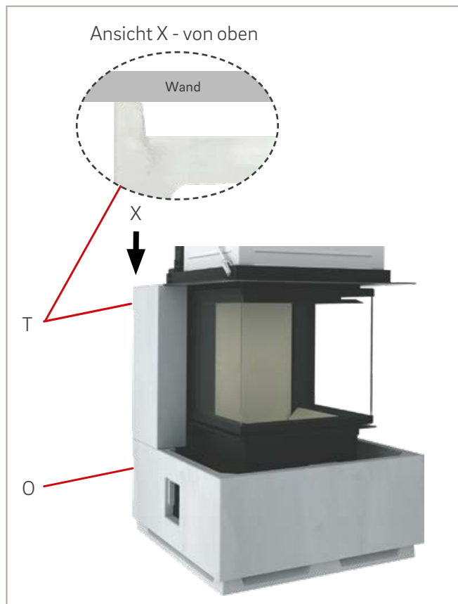
Abb. 40: Seitenteil lang setzen
