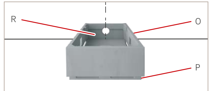
Abb. 16: Unterbauteil setzen
