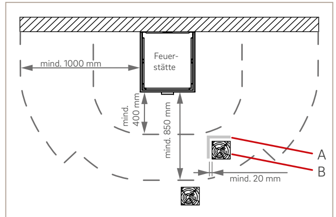
Abb. 75: Schutz von brennbaren Bauteilen im Strahlungsbereich vor der Feuerraumöffnung
