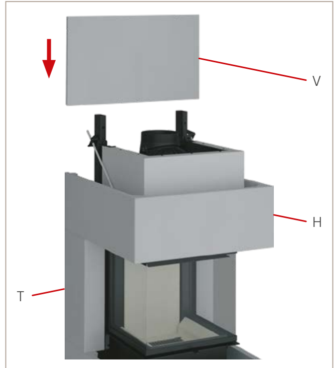
Abb. 43: Rückwand 2 setzen
