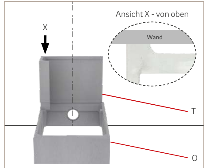
Abb.22: Seitenteil lang setzen
