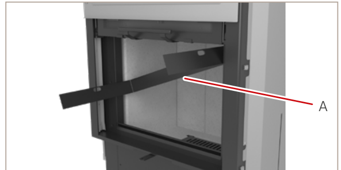
Abb. 63: Halter entnehmen
