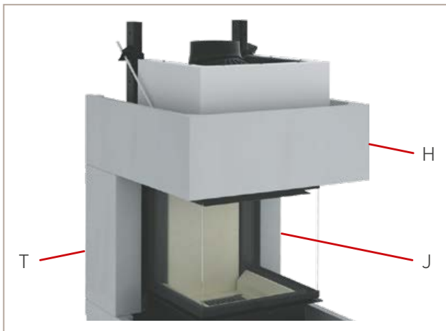
Abb. 42: Oberbauteil 1 setzen
