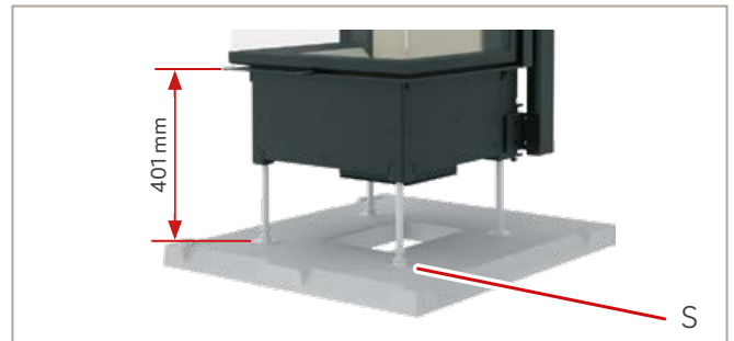
Abb. 30: Stellfüße vorn austauschen
