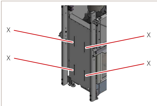
Abb. 25: Position Feststellschrauben am Kamineinsatz
