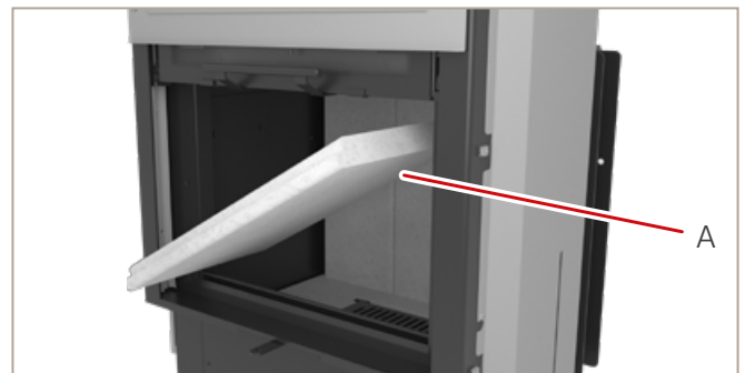
Abb. 64: seitliche Innenauskleidung entnehmen
