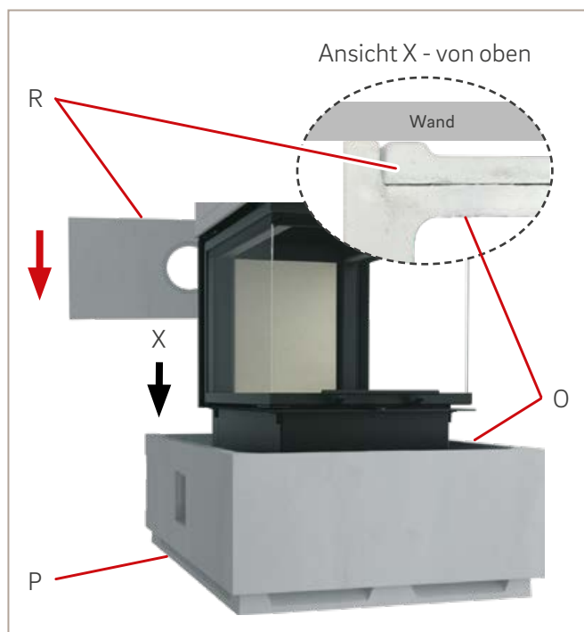
Abb. 39: Rückwand 1 setzen
