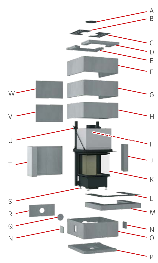
Abb.10: Aufbau am Beispiel S15
