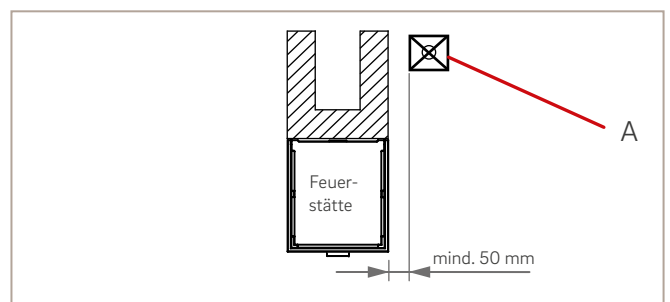
Abb. 76: Schutz und Abstände bei beheizten Flächen
