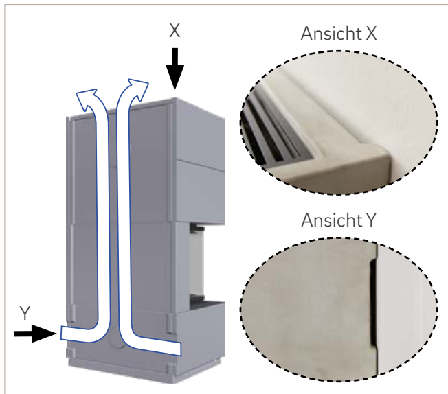
Abb. 77: Aktive Hinterlüftung mit Öffnungen seitlich und oben
