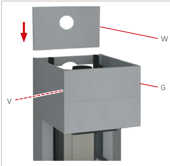
Abb. 45: Rückwand 3 setzen
