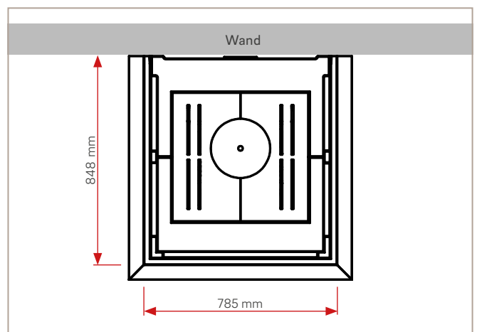
Abb. 12: Estrichaussparung S15 mit Naturstein-Feuertisch
