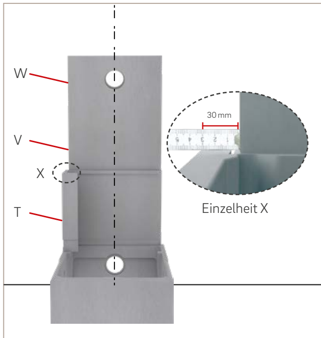
Abb. 23: Rückwand 2 und Rückwand 3 setzen
