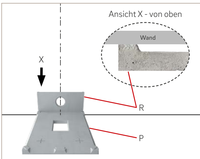
Abb. 15: Rückwand 1 setzen
