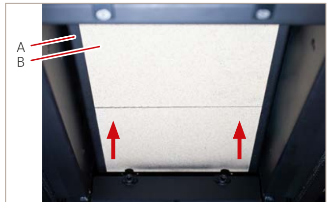
Abb. 69: Prallplattenteile mit Prallplattenhalter
