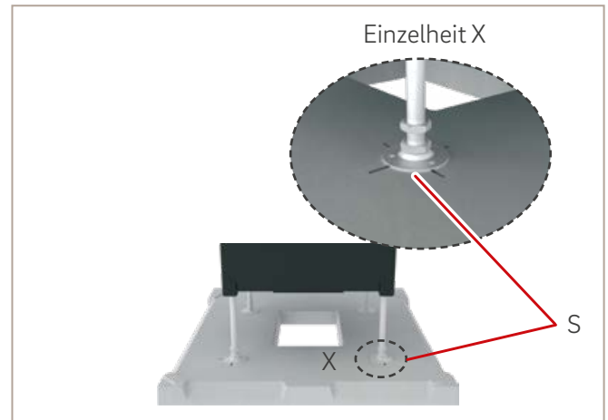
Abb. 27: Kamineinsatz positionieren
