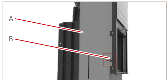
Abb. 59: Demontage Gewichtsschachtabdeckungen
