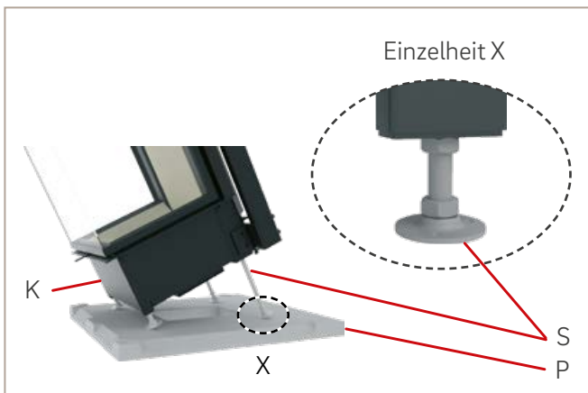
Abb. 29: Kamineinsatz nach vorn kippen und Stellfüße einstellen
