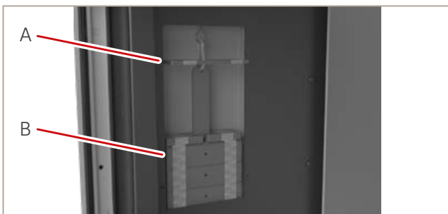
Abb. 68: Ausgleichsgewicht entnehmen
