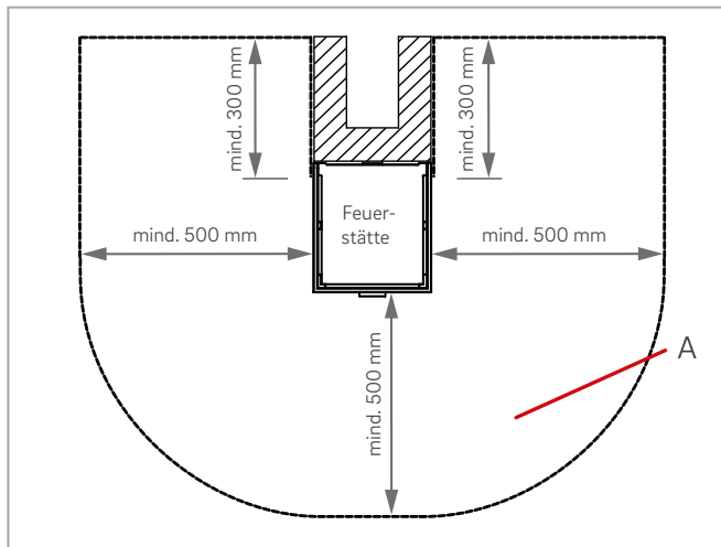
Abb. 74: Belag aus nicht brennbaren Baustoffen im Bereich vor der Feuerraumöffnung
