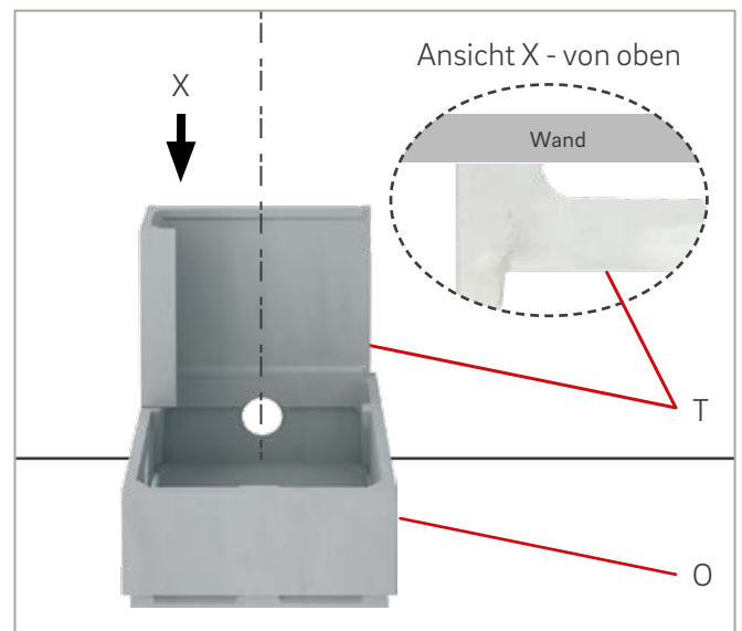
Abb. 17: Seitenteil lang setzen
