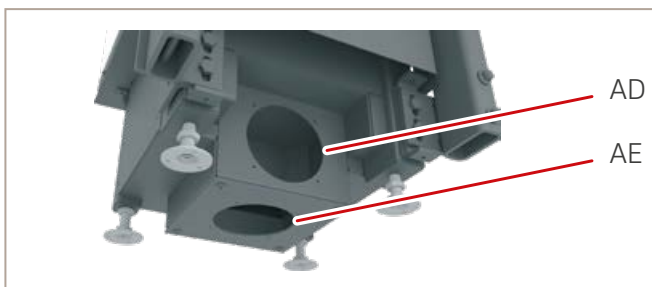
Abb. 34: Anschlussöffnungen Verbrennungszuluft
