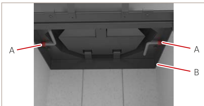
Abb. 62: Befestigungsschrauben lösen
