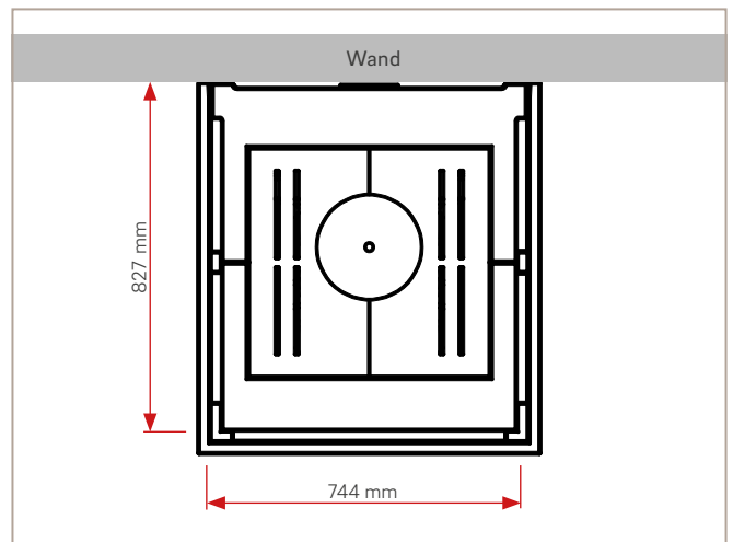
Abb. 11: Estrichaussparung S15
