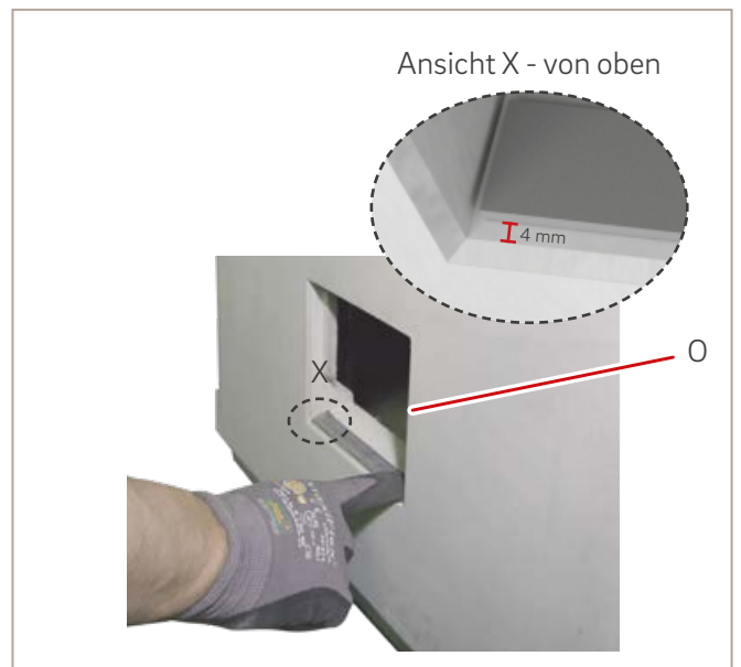
Abb. 48: Revision Dichtungsband 140 mm unten einkleben
