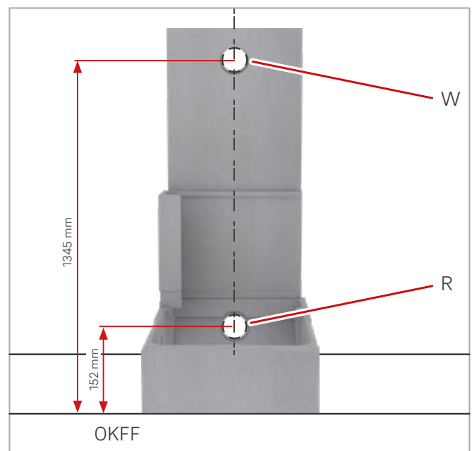
Abb. 24: Anschlüsse an der Zimmerwand anzeichnen und bohren
