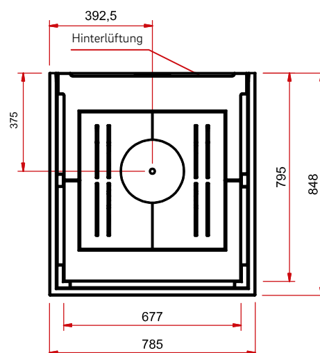
Draufsicht M 1:20
