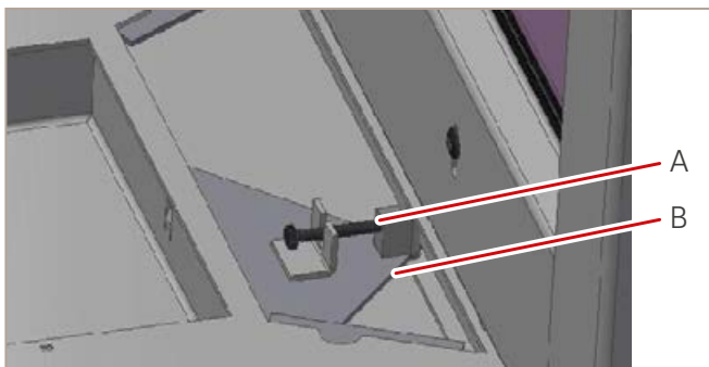
Abb. 58: Befestigungsschraube lösen
