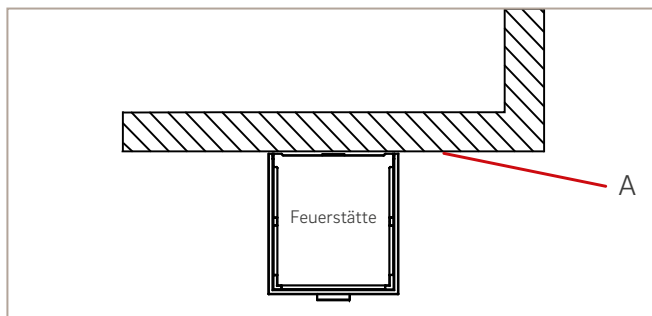
Abb. 78: Schutz und Abstände zur Wand
