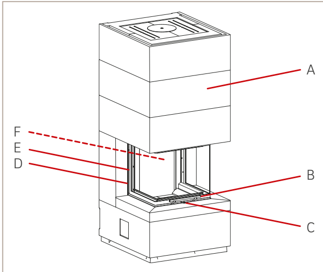
Abb.2: Abbildung S15
