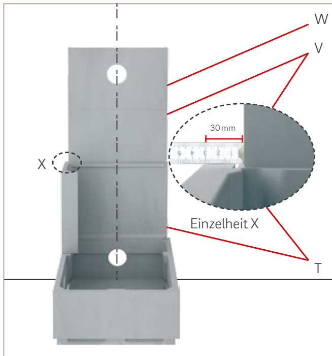
Abb. 18: Rückwand 2 und Rückwand 3 setzen
