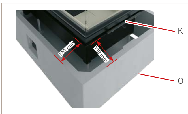
Abb. 37: Kamineinsatz ausrichten
