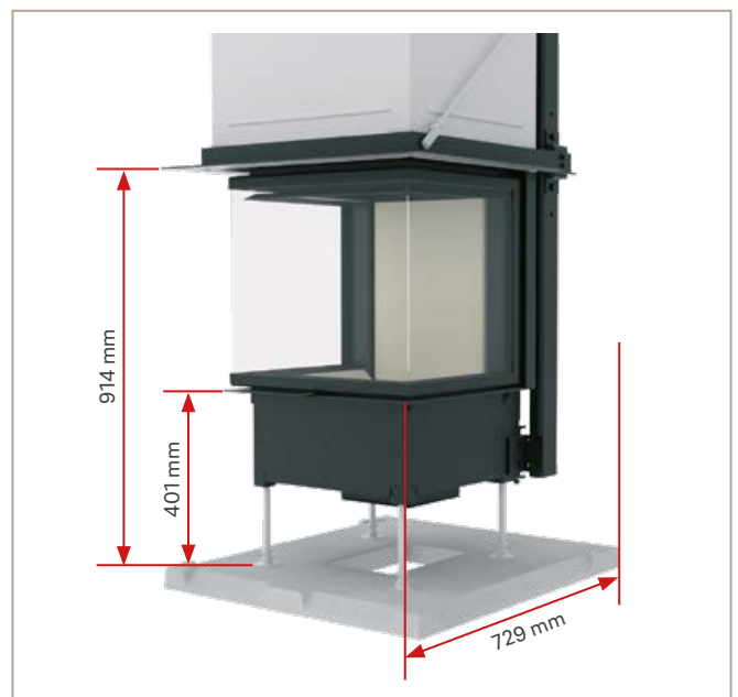
Abb. 31: Höhe und Abstand zur Wand einstellen
